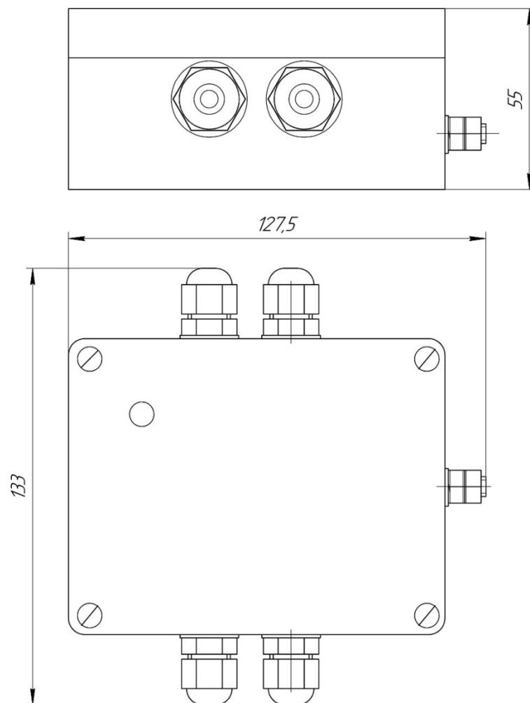
Рисунок 1 - Габаритный чертеж корпуса
